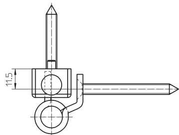
SIKU RB 5015 3D - Bohrmaß 11,5 mm - Drilling dimension 11,5 mm
