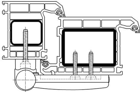
Сечение
