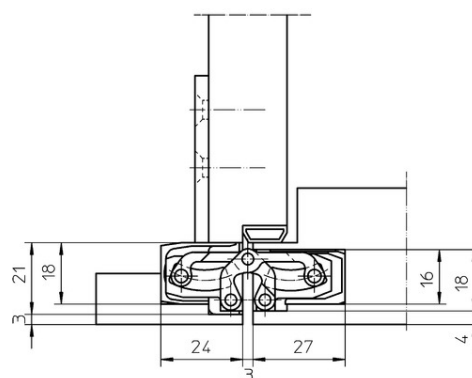
охватывающая дверная коробка
