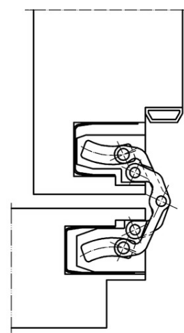
блочная дверная коробка 180°
