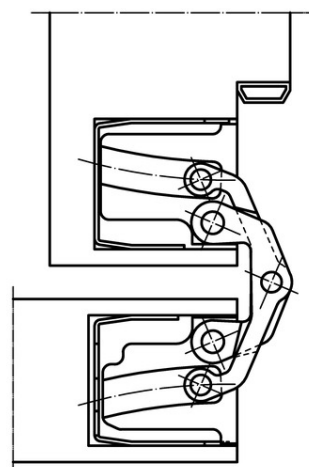
блочная дверная коробка 180°
