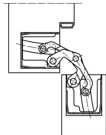
блочная дверная коробка 90°
