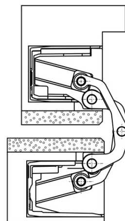
блочная дверная коробка 180°
