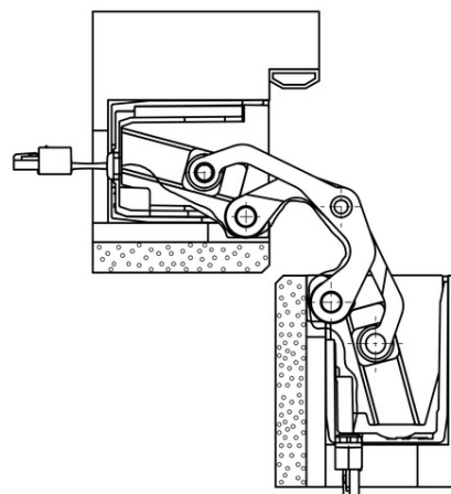
блочная дверная коробка 90°
