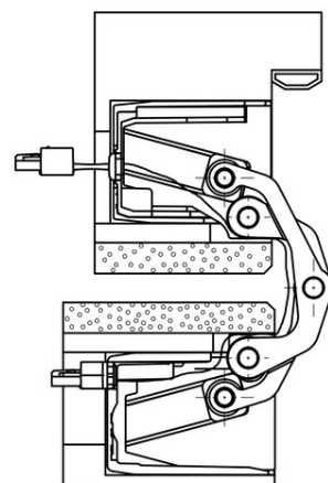
блочная дверная коробка 180°
