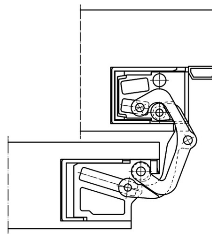
блочная дверная коробка 180°
