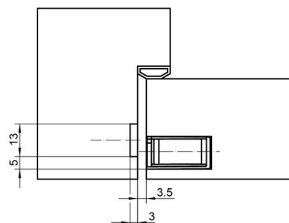
Разрез без фальца
