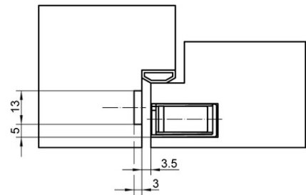
Сечение исполнение заподлицо с фальцем
