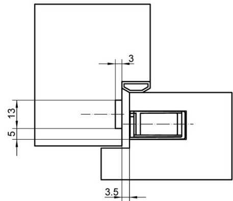
Разрез с фальцем
