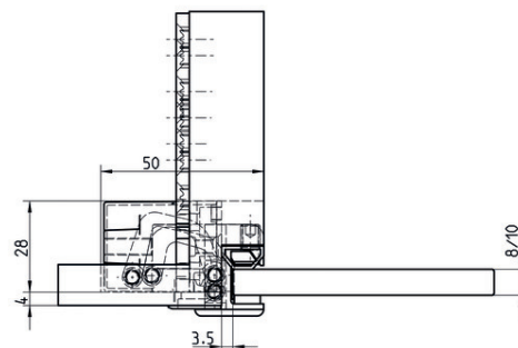
охватывающая дверная коробка
