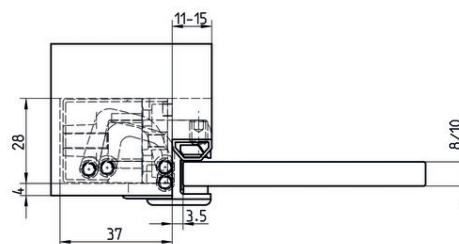
блочная дверная коробка
