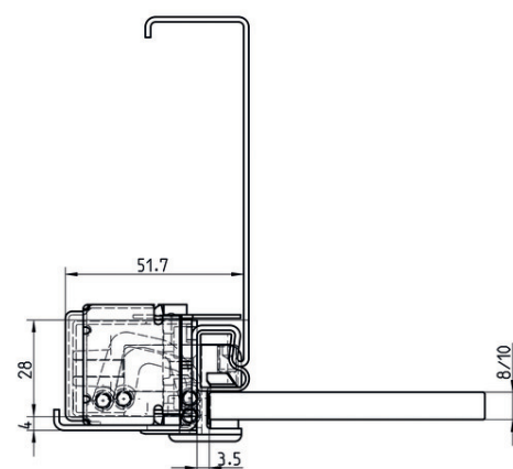
стальная дверная коробка
