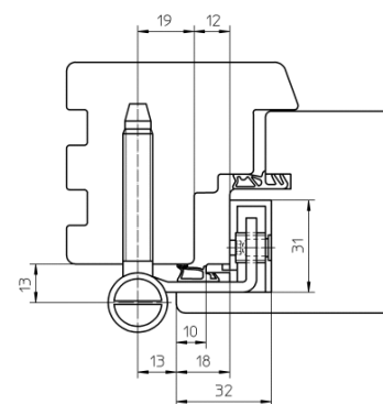
фальц 18 мм (головная часть уплотнителя 10 мм)
