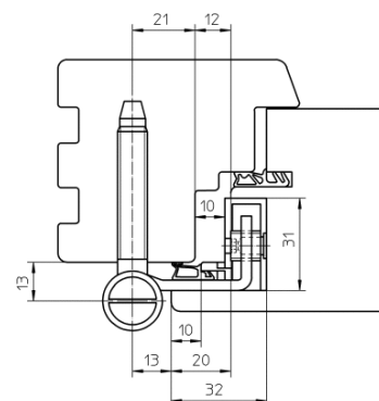
фальц 20 мм (головная часть уплотнителя 10 мм)
