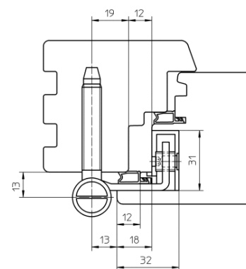
фальц 18 мм (головная часть уплотнителя 12 мм)
