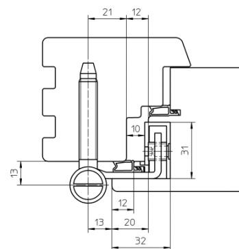
фальц 20 мм (головная часть уплотнителя 12 мм)
