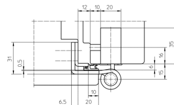
фальц 20 мм (головная часть уплотнителя 10 мм)
